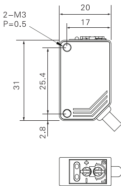
NPN Output
